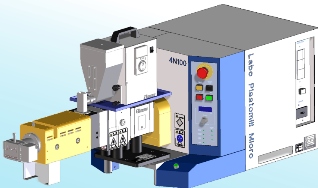
▼押出機仕様
